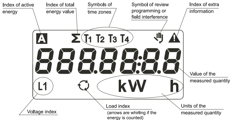
Fig. 4 LCD display
