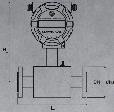
FLANGE (EN 1092)
