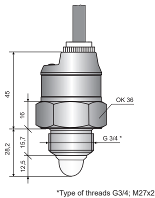
RFLS-35_-2-G3/4
